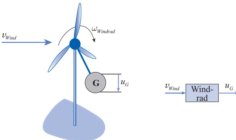
Bild 2.2 System Windrad
