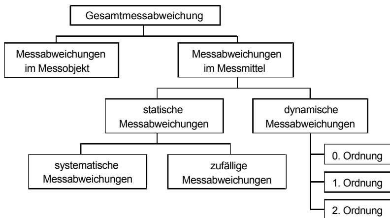
Bild 1.14 Überblick und Zusammenhang der Messabweichungen
