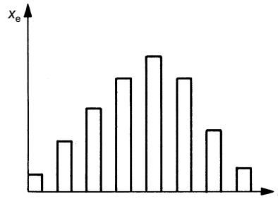
Bild 1.6 Amplituden- und zeitquantisiertes Signal
