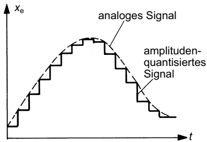
Bild 1.5 Amplitudenquantisiertes Signal
