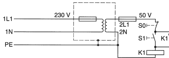
Bild 2.21 Schaltung für Funktionskleinspannung
