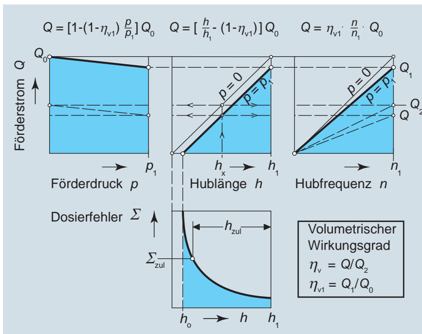
Bild 3.2: Dosierpumpen-Kennlinien ( Q_0 Förderstrom bei p \approx 0 , h = h_p , n = n_p ; Q_1 Förderstrom bei p = p_p , h = h_p , n = n_p ; Q_2 Förderstrom bei p = p_p , h = h_x , n = n_p )
